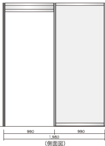
(側面図)
